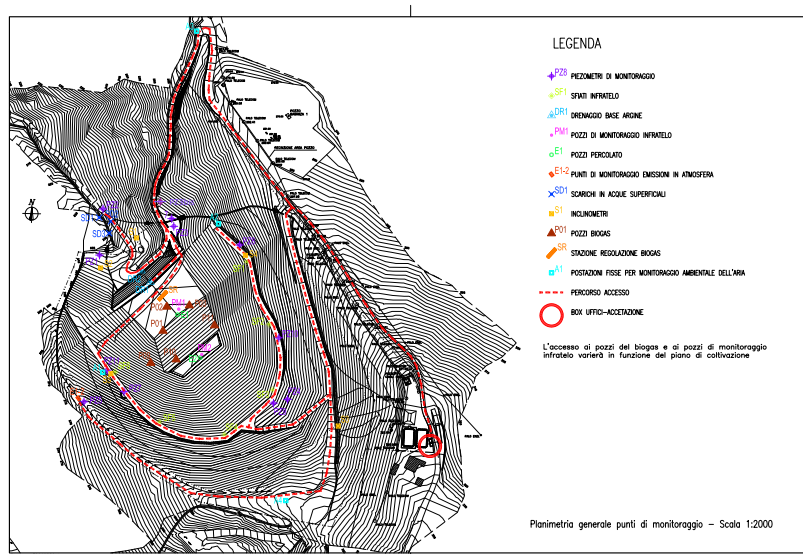
Figura 13-9 Schema della rete di controllo piezometrico della discarica Palladio Team Fornovo S.r.l.
