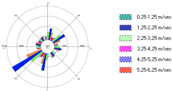
Figura 13-3 Rose dei venti annuali del periodo 2024 – 2025 presso la discarica Palladio Team Fornovo S.r.l.
