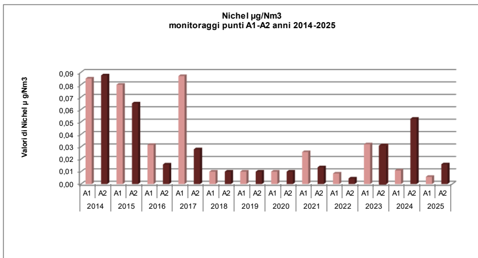
Figura 13-7 Nichel nell'aria (2014-2025)
