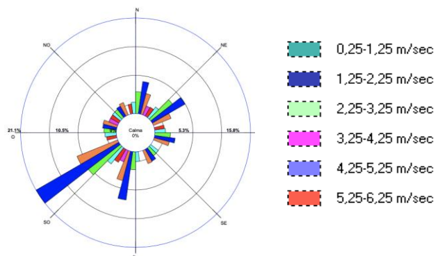
Figura 13-3 Rose dei venti annuali del periodo 2023 – 2024 presso la discarica Palladio Team Forno S.r.l.
