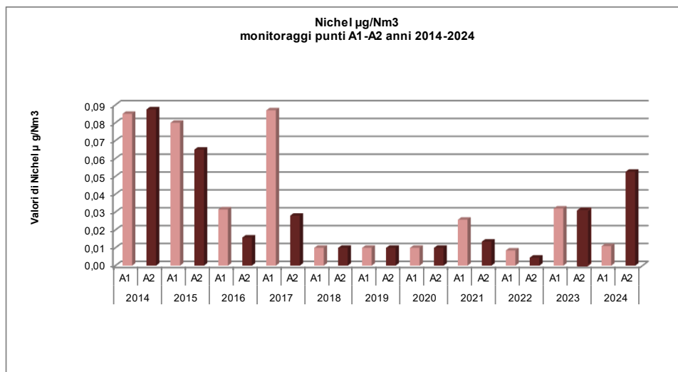
Figura 13-7 Nichel nell'aria (2014-2024)
