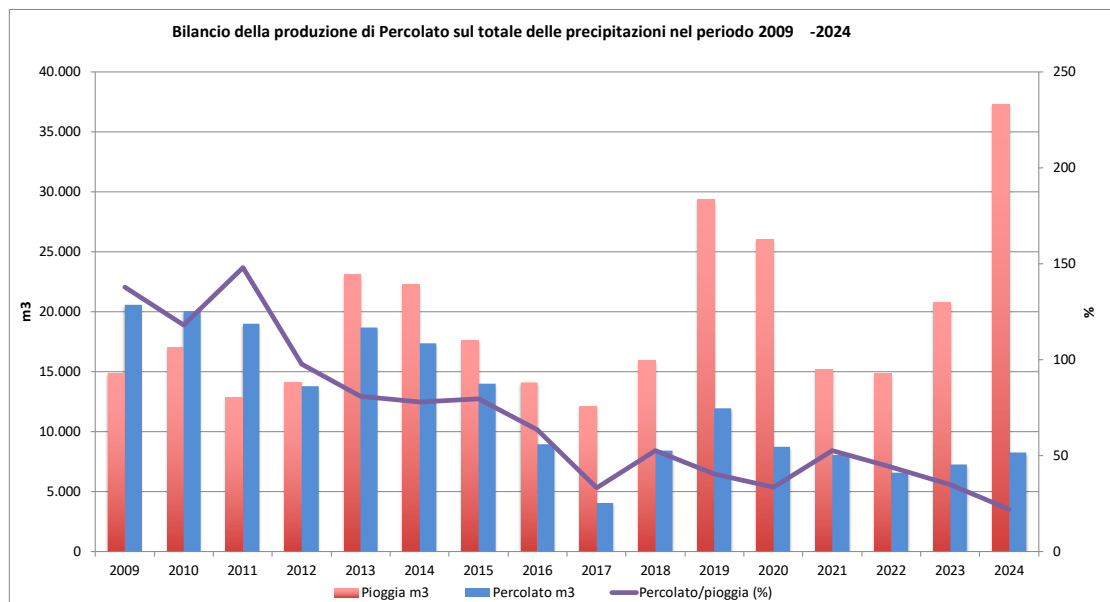
Figura 13-13 Bilancio idrologico
