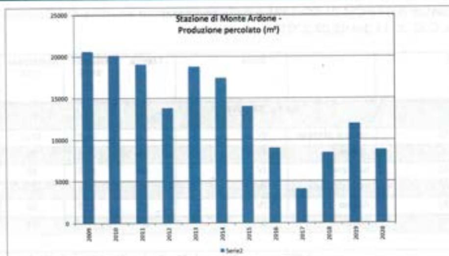
Figura 15-1 - Quantità di Percolato Prodotto nel periodo 2009-2020
