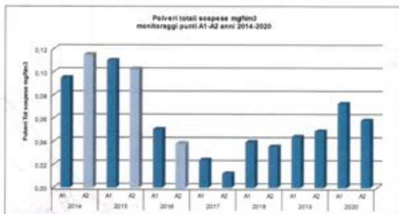
Figura 15-7 - Andamento nel tempo delle concentrazioni di PTS valori espressi in mg/Nm³
