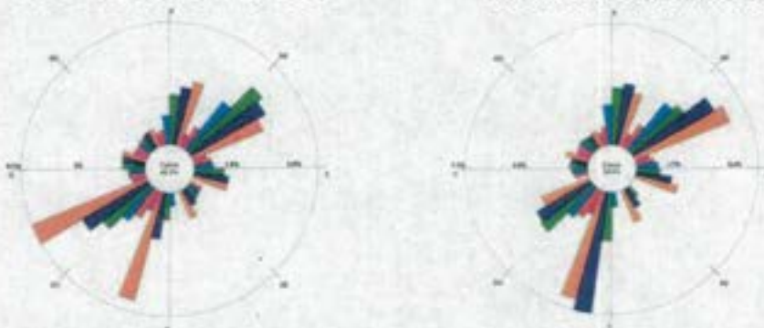
Figura 15-3 Rose dei venti annuali del periodo 2018 - 2021 (3) presso la discarica Palladio Team Fornovo S.r.l.
