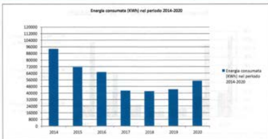
Figura 15-22 Consumi totali di energia elettrica
