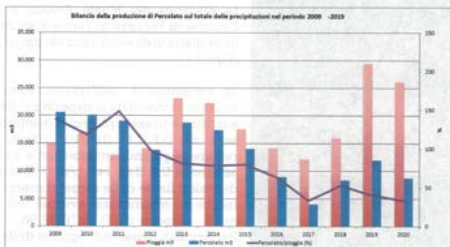
Figura 15-15 Bilancio idrologico
