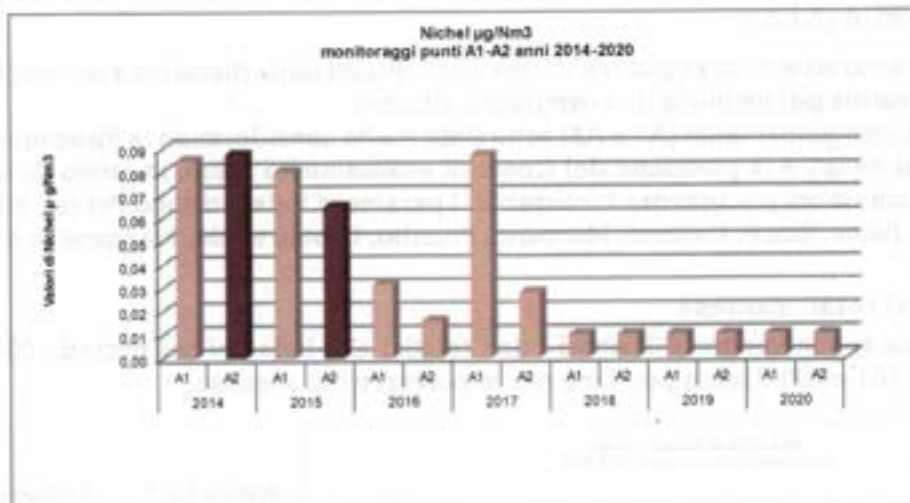
Figura 15-9 Nichel nell'aria (2014-2020)
